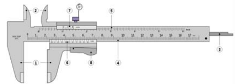
Gambar 4. Bagian – bagian jangka sorong [6]
