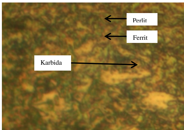
Gambar 5. Hasil Struktur Mikro Baja S45C dengan Holding Time 30 Menit SAE 10W-30
