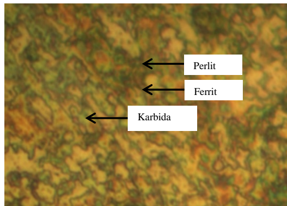
Gambar 10. Hasil Struktur Mikro Baja S45C dengan Holding Time 50 Menit SAE 20W-50
