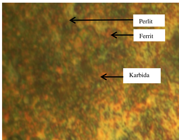
Gambar 7. Hasil Struktur Mikro Baja S45C dengan Holding Time 30 Menit SAE 20W-50
