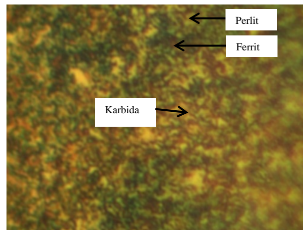
Gambar 4. Hasil Struktur Mikro Baja S45C sebelum Heat Treatment
