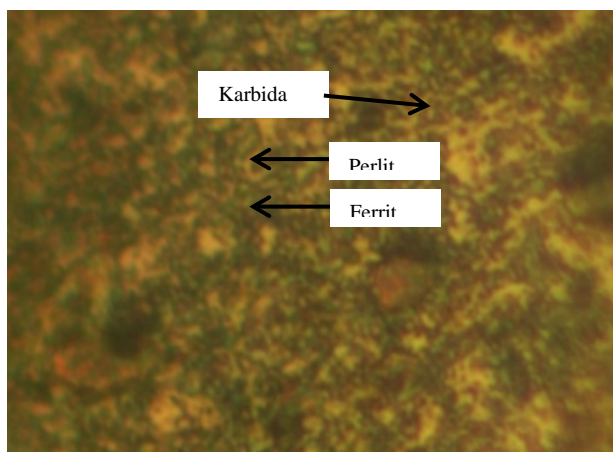
Gambar 6. Hasil Struktur Mikro Baja S45C dengan Holding Time 30 Menit SAE 15W-40
