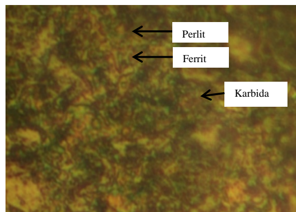
Gambar 9. Hasil Struktur Mikro Baja S45C dengan Holding Time 50 Menit SAE 15W-40
